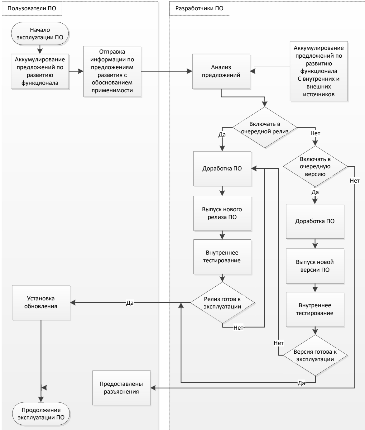
Рисунок 2. Процесс развития ПО
