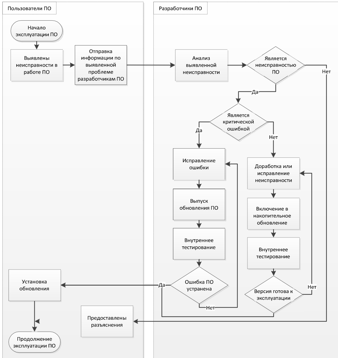
Рисунок 1. Процесс устранения неисправностей ПО
